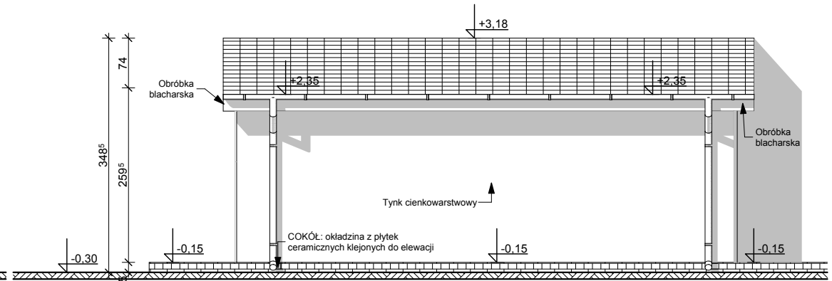
ELEWACJA BOCZNA
