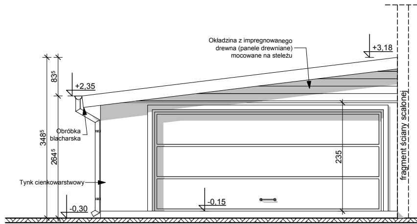
ELEWACJA FRONTOWA
