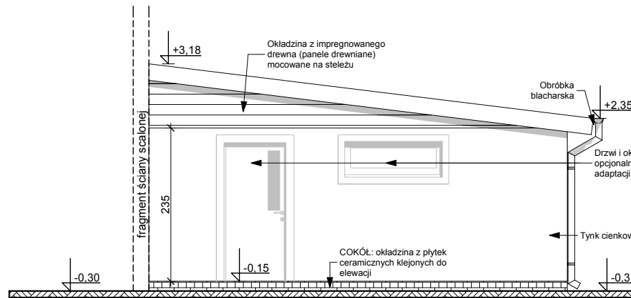
ELEWACJA OGRODOWA
